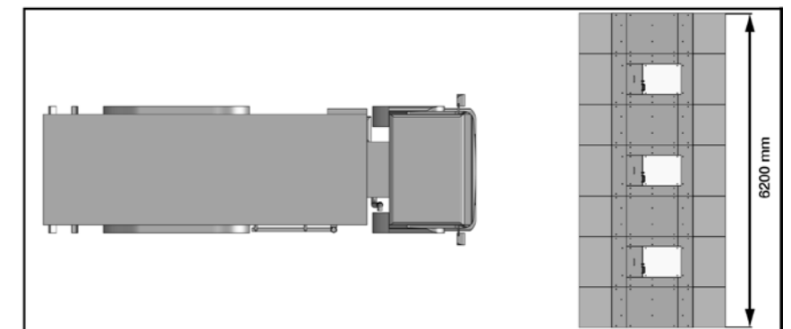
Konfiguration mit drei Modulen und Sperrelement sowie vier Modulen für den Fußgängerdurchgang
